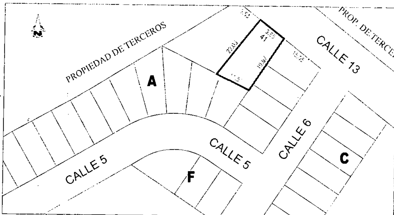
LOTIZACION
