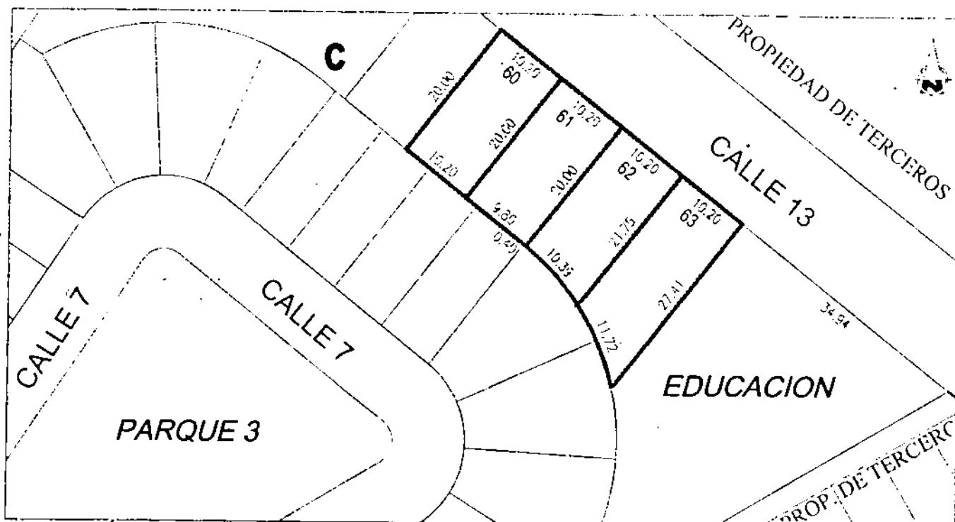
LOTIZACIÓN
