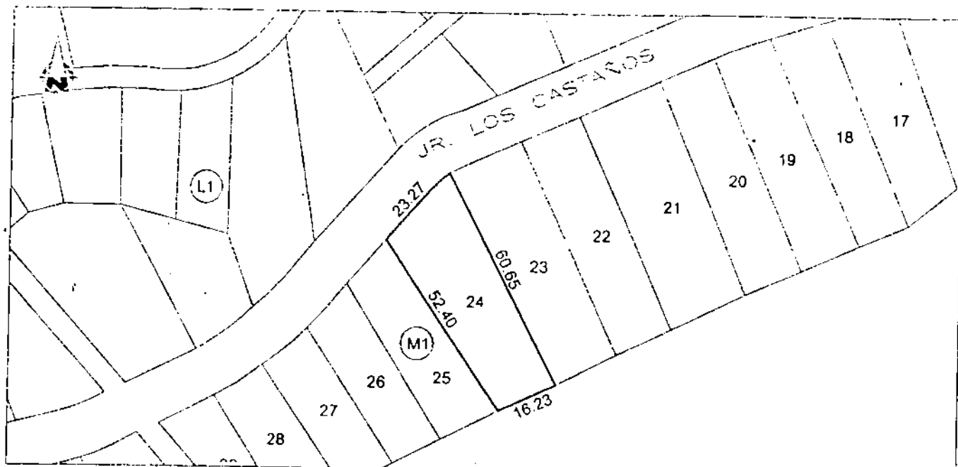
LOTIZACIÓN
