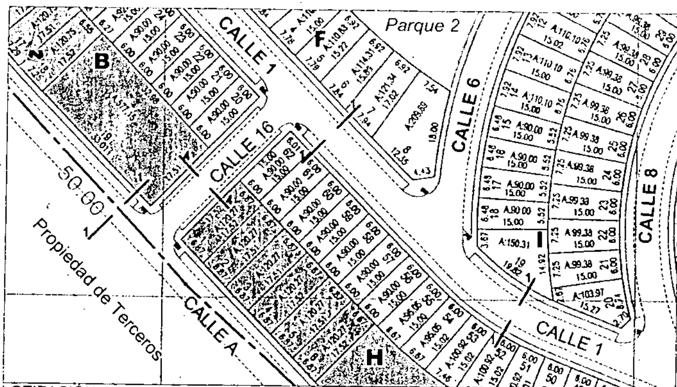
LOTIZACIÓN
